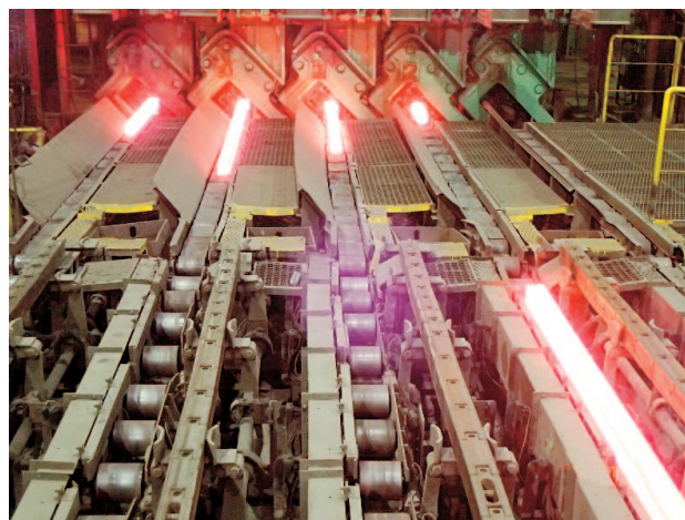
視察した処分業者事業所での電気炉を用いた溶融処理 および建築に使用する鉄筋材の製造の様子
