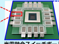
光電融合スイッチボード (3.2 Tbit/s × 16台)
