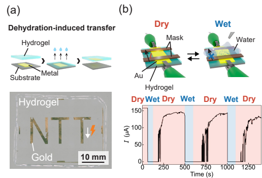
(a) 金属薄膜は任意のパターンで接着させることができる (b) ゲルの完全乾燥時に転写した金属は、周囲の水分に反応したゲルの膨潤・脱膨潤で導電性を変える配線になる
