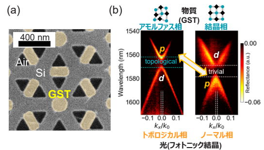
(a) 作製したトポロジカルフォトニック結晶のSEM写真。シリコンフォトニック結晶の構造上にナノメートルスケールの小さなGSTが高い位置精度で装荷されている(b)角度分解反射分光により測定した光バンド構造。物質相転移に伴う上下のバンドの明るさの変化によりトポロジカル相転移が示されている
