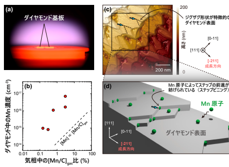
(a) マイクロ波プラズマCVD法によるダイヤモンド成長の様子 (b) 気相中の[Mn/C]比とダイヤモンド中のMn濃度の関係 (c) Mnドーピングダイヤモンド(111)薄膜表面の原子間力顕微鏡像 (d) Mnドーピングダイヤモンド(111)薄膜の成長機構の模式図
