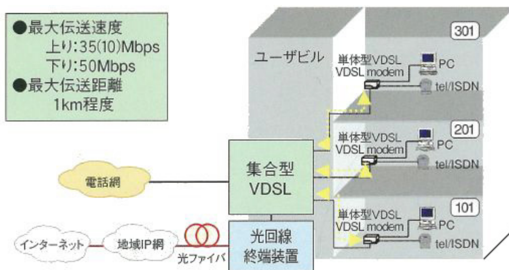
図 構内系 VDSL 装置
