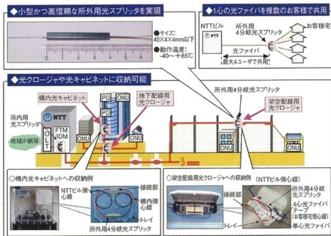
図 所外用光スプリッタとその収容技術
